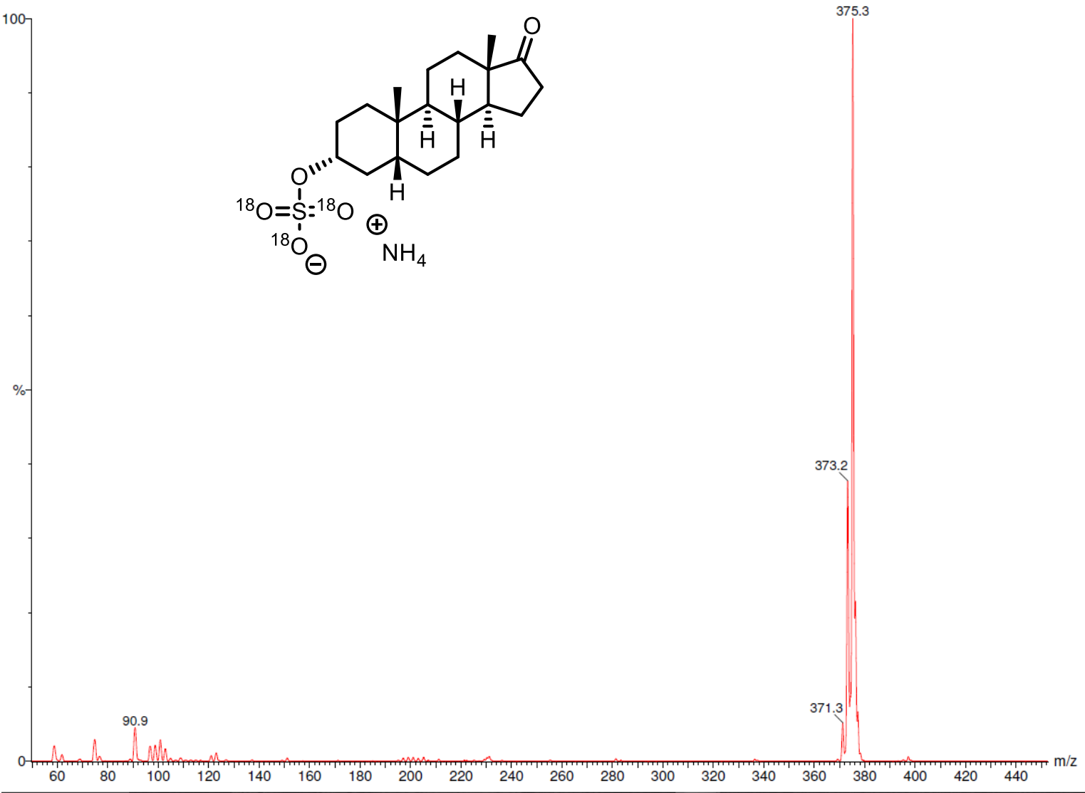
Etiochocanolone 3-[ 18 O 3 ]-sulfate, ammonium salt LRMS
