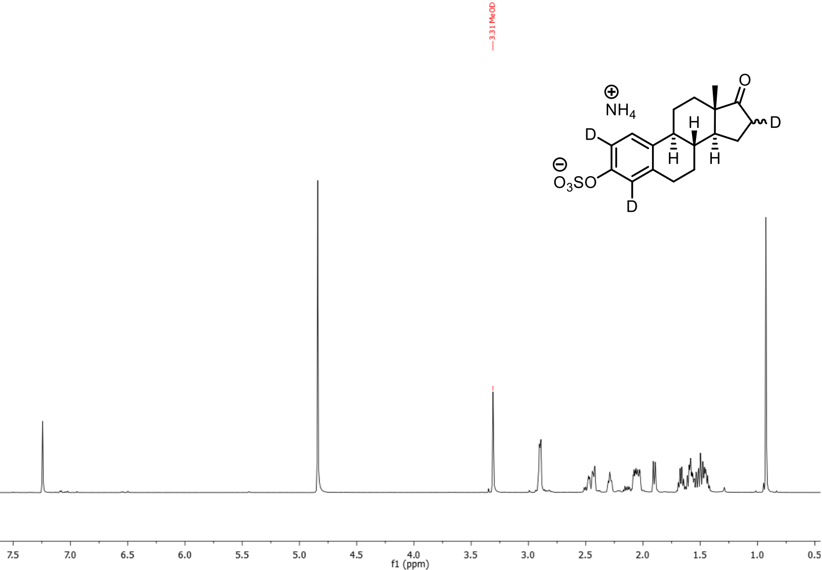
2,4,16- d 3 -Estrone 3-sufate 1 H NMR 400 MHz, CD 3 OD
