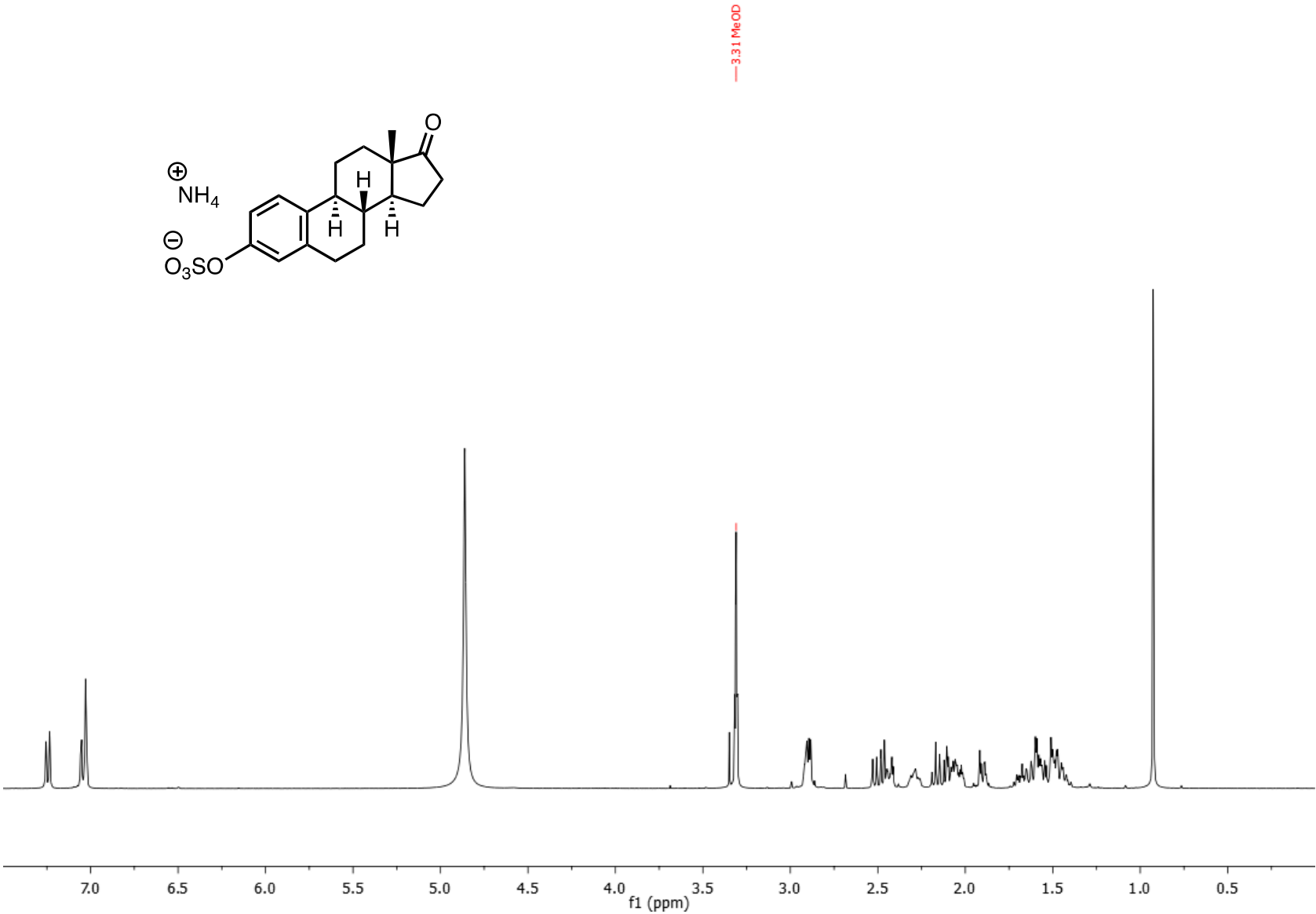
Estrone 3-sulfate, ammonium salt 1 H NMR 400 MHz, CD 3 OD
