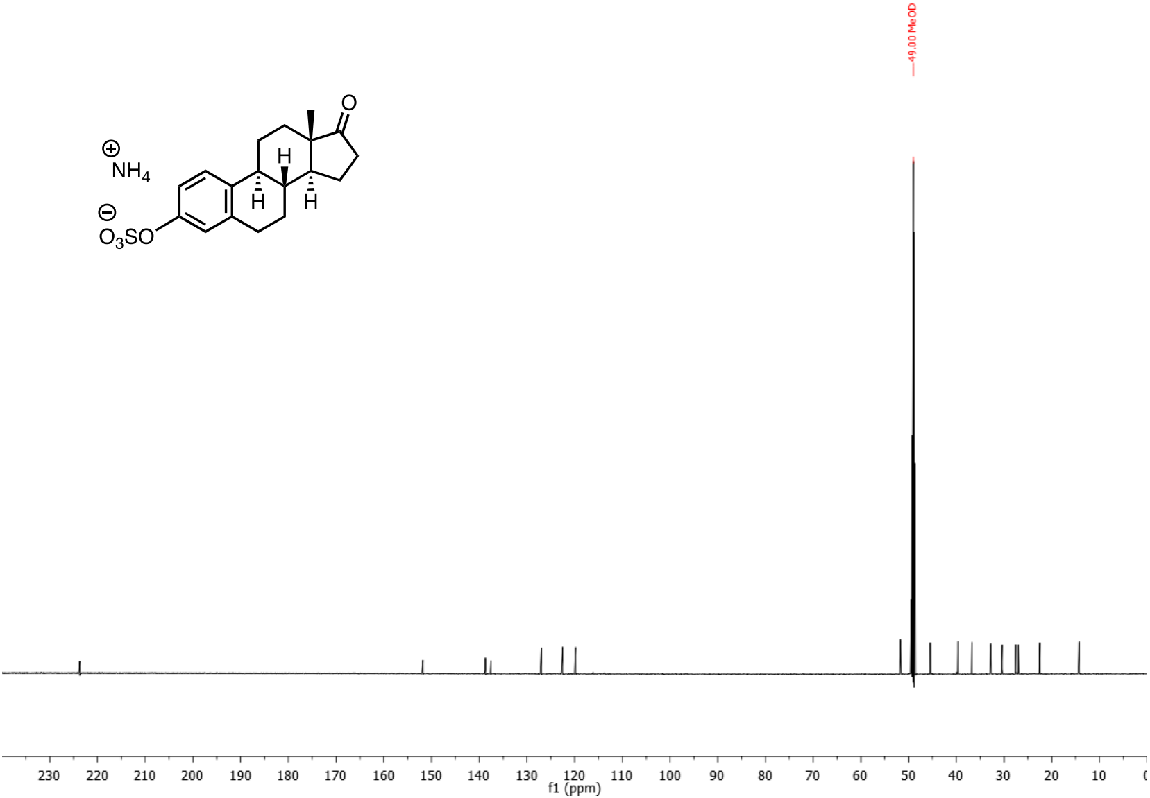
Estrone 3-sulfate, ammonium salt 13 C NMR 151 MHz, CD 3 OD
