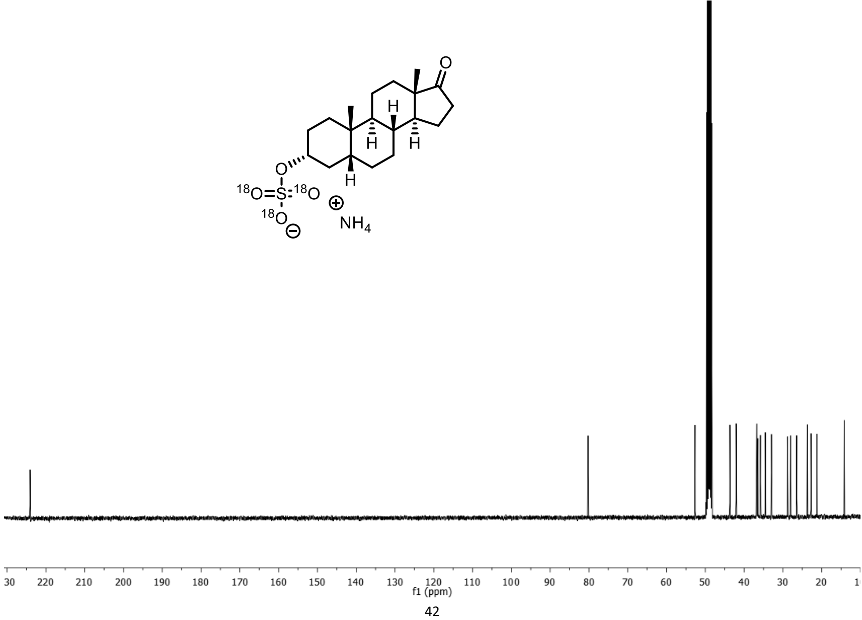
Etiochocanolone 3[ 18 O 3 ]-sulfate, ammonium salt 13 C NMR 101 MHz, CD 3 OD
