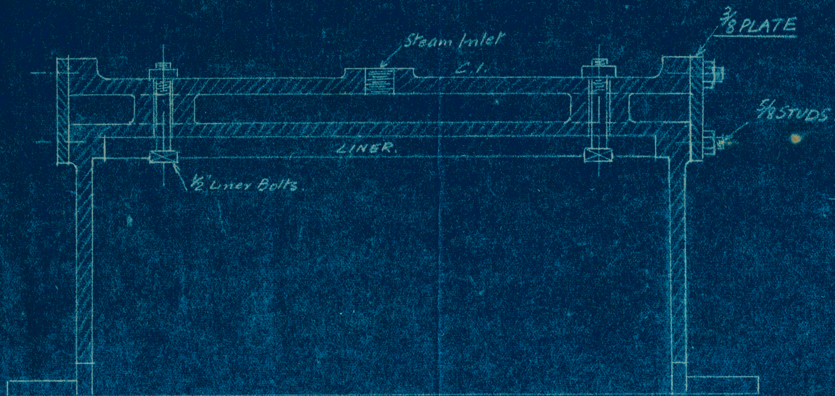
ELEVATION AA. SECTIONAL
